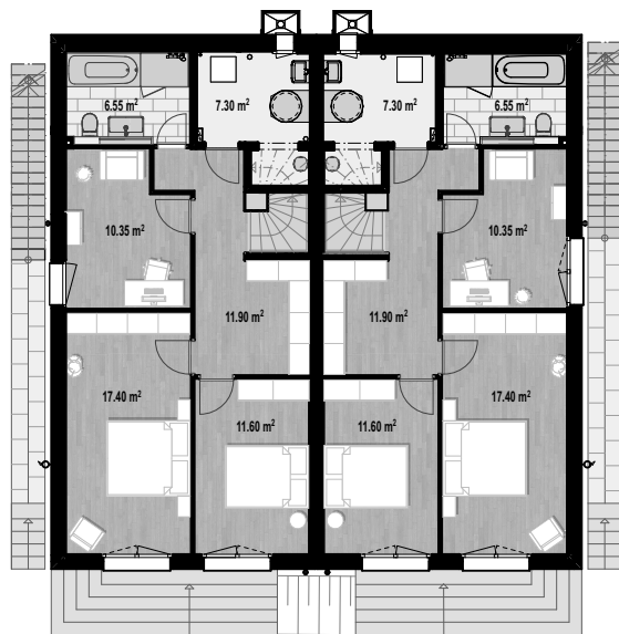
Untergeschoss Mst. 1:200
